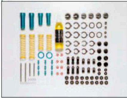
Alu-Öldruckstoßdämpfer-Set
